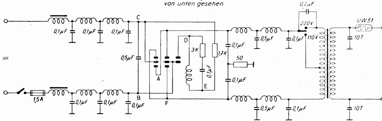
Sockelschaltung f Vibrator von unten gesehen
